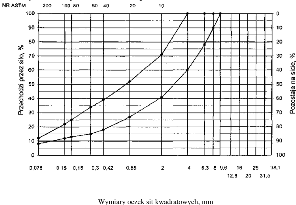
Rys. 3. Krzywe graniczne uziarnienia mieszanki mineralnej BA od 0 do 8mm, od 0 do 6,3 mm do warstwy ścieralnej nawierzchni drogi o obciążeniu ruchem nawierzchni drogi o obciążeniu ruchem KR1
