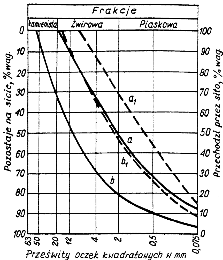
Rysunek 1. Obszar uziarnienia optymalnych mieszank zwirowych
