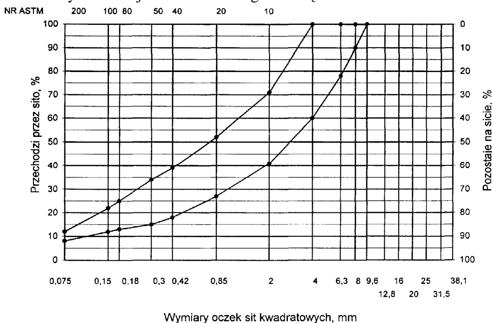
Rys. 3. Krzywe graniczne uziarnienia mieszanki mineralnej BA od 0 do 8mm, od 0 do 6,3 mm do warstwy ścieralnej nawierzchni drogi o obciążeniu ruchem KR1
