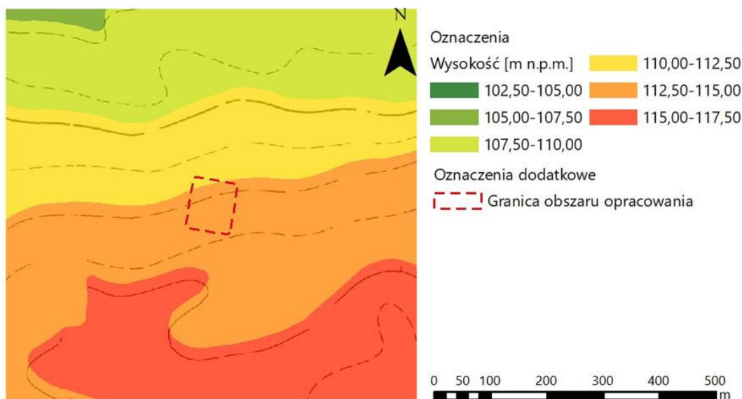
Rys. 4 Ukształtowanie terenu
