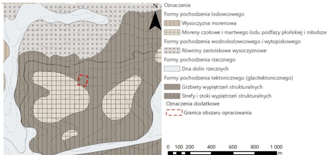
Rys. 5 Formy geomorfologiczne
