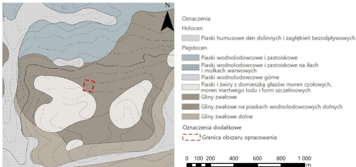
Rys. 3 Utwory geologiczne
